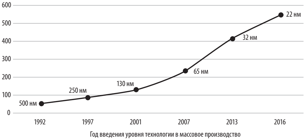
Рисунок 5. Средняя стоимость завода по производству наносхем, млн долл.
